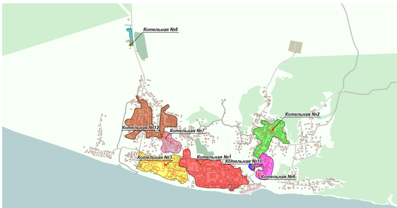
Рисунок 4 – Зоны действия источников централизованного теплоснабжения МП МО Октябрьский район «ОКС» на территории поселения
