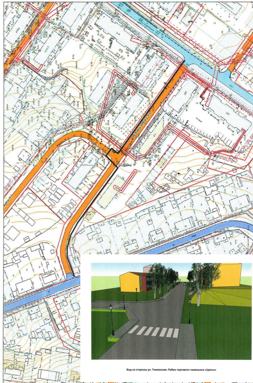
Схема размещения тротуара на плане территории с.п.Уньютан
